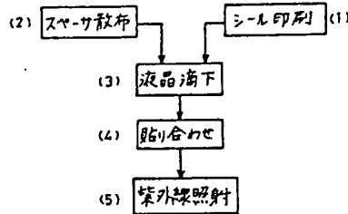
本発明に係る液晶ディスプレイの製造工程を示す流れ図 第1図
